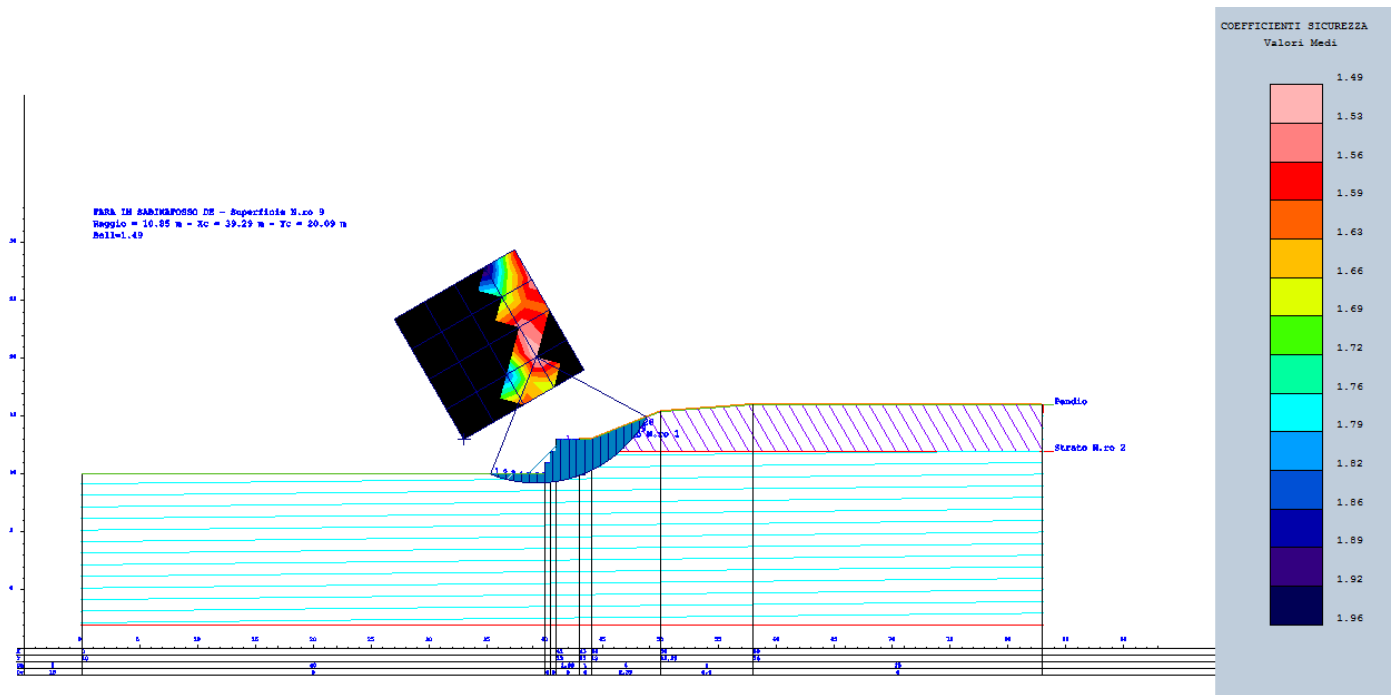
Verifica stabilità globale pendio Muro 1
