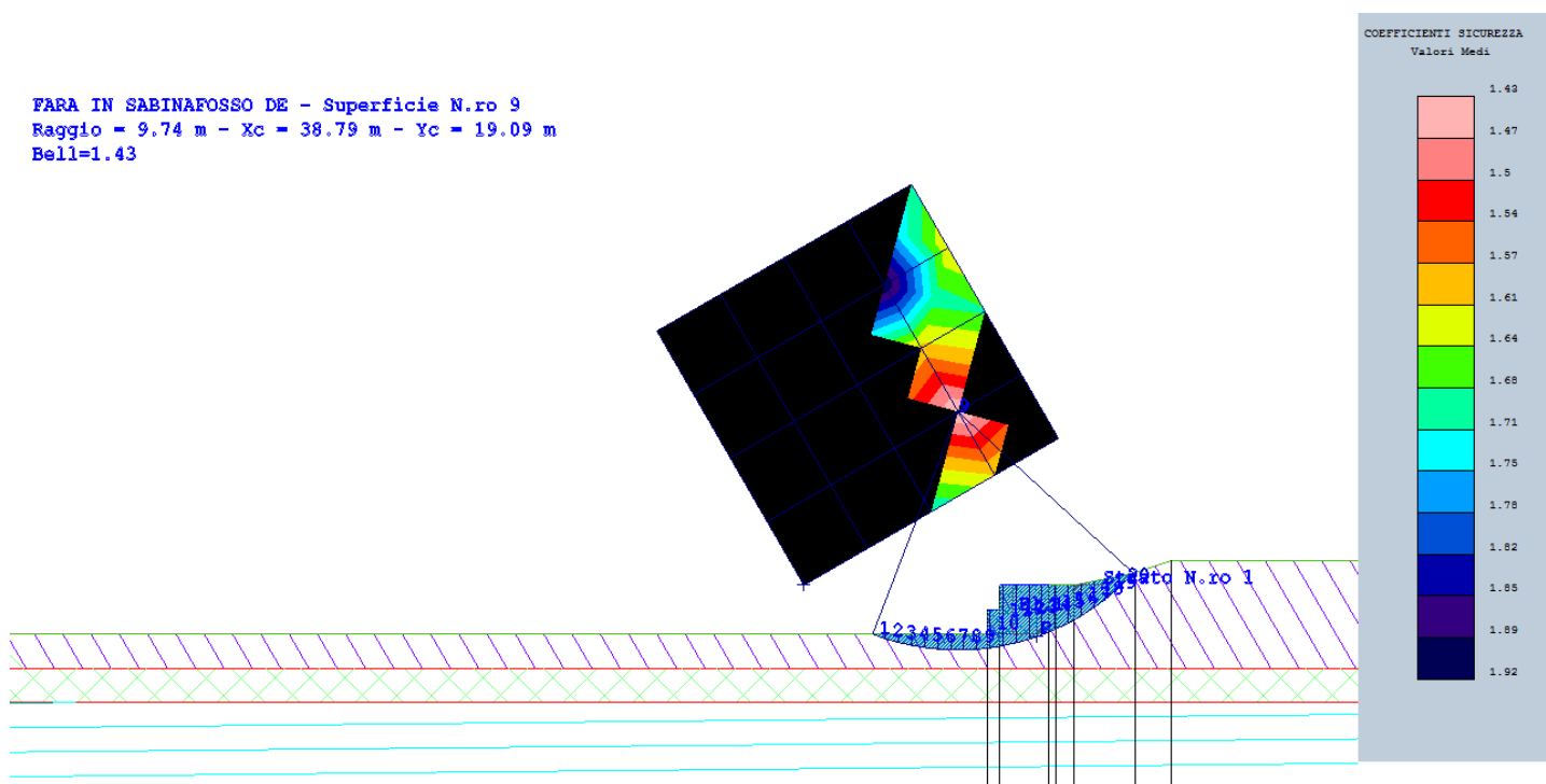
Verifica stabilità globale pendio Muro 2
